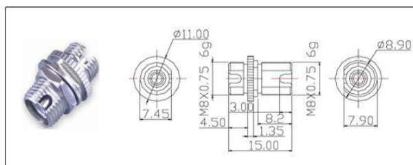
Figure4. FC D Adaptor
